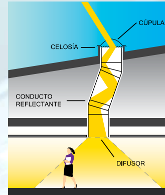
Tubo de Luz Solar
